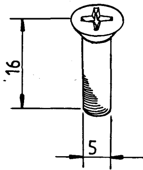
Senkschraube M 5 x 16
