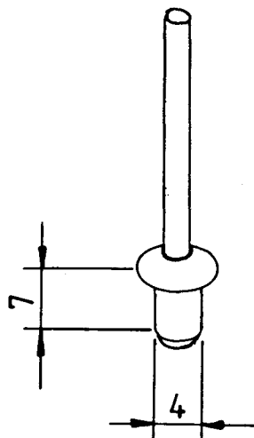
Blindniet 4,0 x 7
