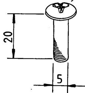
Linsenschraube M 5 x 20
